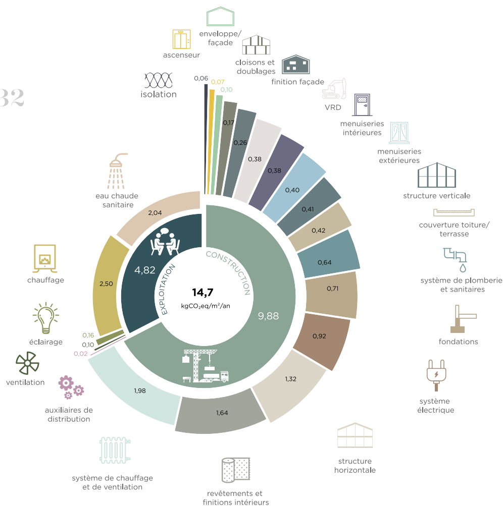
Distribution de l'empreinte carbone par lots Opération d'Habitat collectif 38 logements . R+3 . 3 300m² SDP
